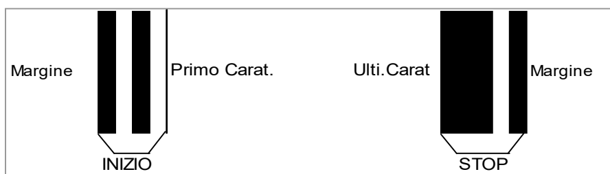
Figura 5.3.2.1.2-1. Barre iniziali e finali
