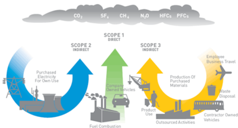
Esemplificazione degli Scope previsti dal GHG Protocol
