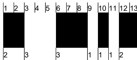
Figura 5.4.3.1-3. Carattere Stop del Simbolo GS1-128
