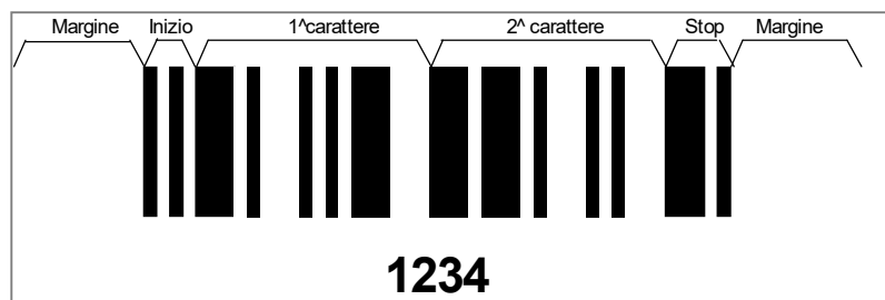
Figura 5.3.2.1.2-2. Simbolo ITF-14 compresi i margini
