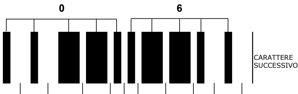
Figura 5.3.2.1.1-3. ITF-14 coppie di caratteri che codificano le cifre 03 e 67
