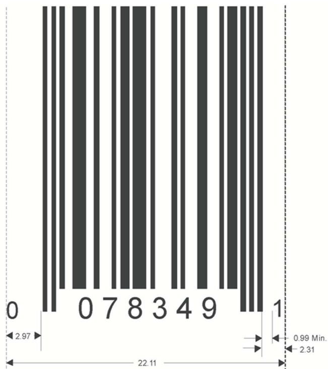
Figura 5.2.6.6-4. Simbolo UPC-E
