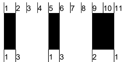
Figura 5.4.3.1-3. Carattere Stop del Simbolo GS1-128
