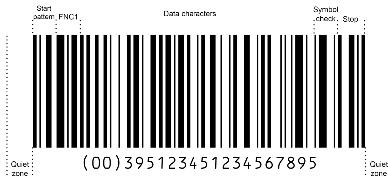
Figura 5.4.2-1. Formato generale del simbolo GS1-128
