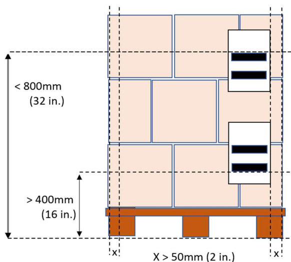
Figura 6.7.1.1-1. Posizionamento del simbolo sui pallet
